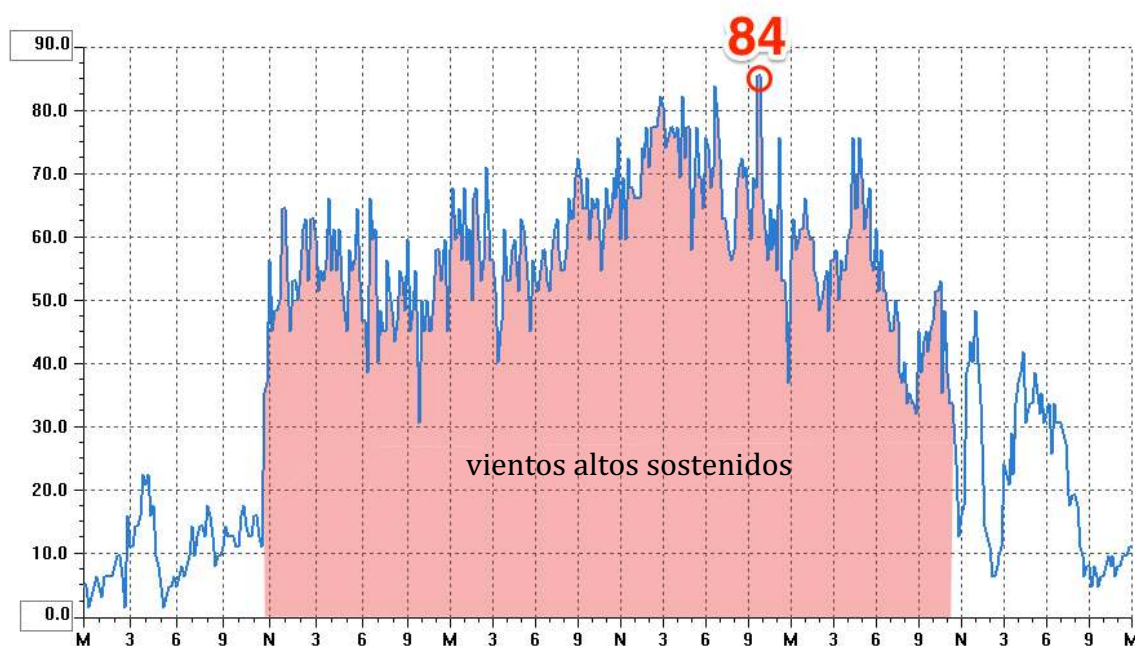
Ráfagas de viento registradas por la estación meteorológica de MASSAMAGRELL entre el 19 y el 21/01/20 (en km/h)
