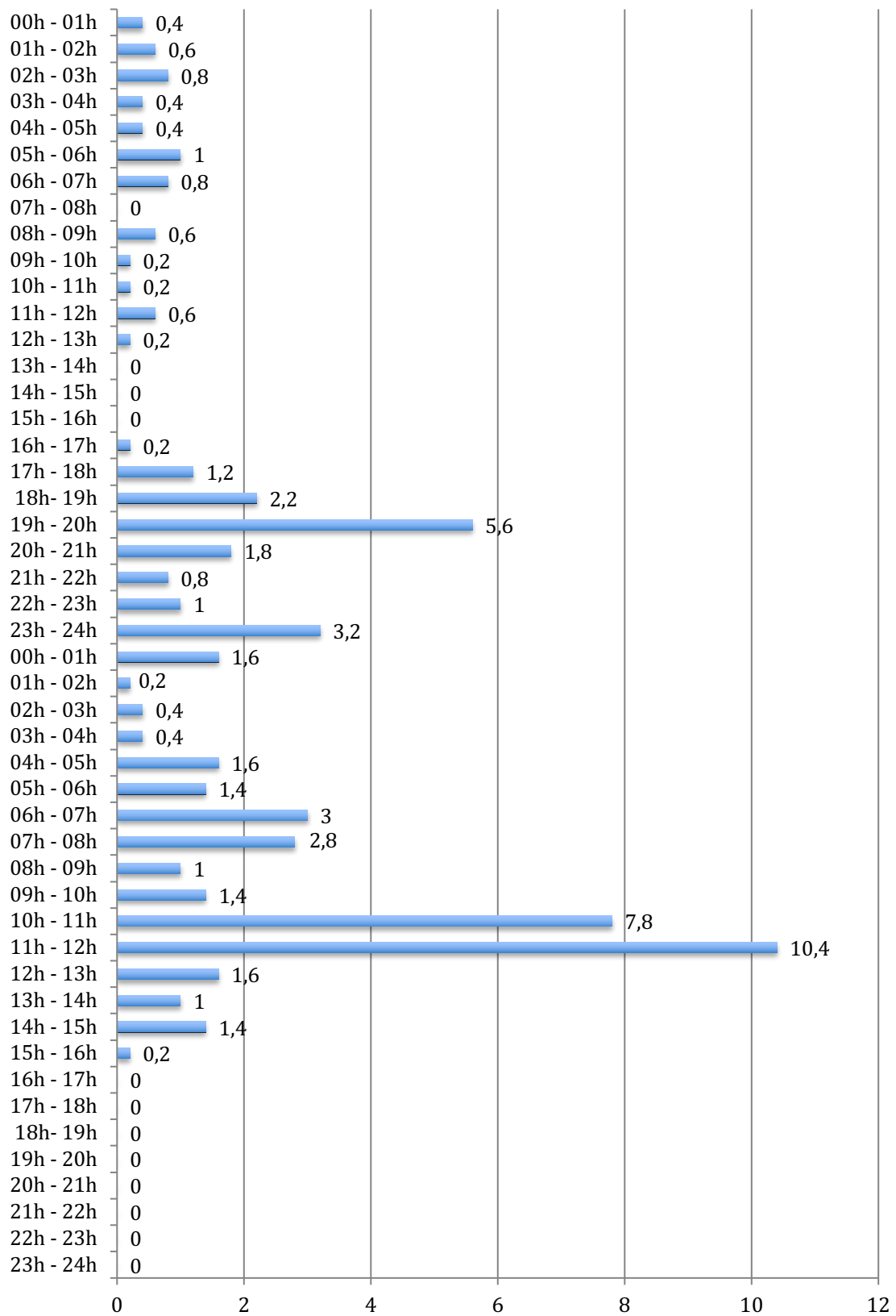
Cantidades de lluvia registradas por horas en MASSAMAGRELL los días 20 y 21 de enero de 2020 (en l/m²)
